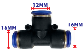
UNIÃO "T" PARA EMENDA C/ REDUÇÃO 16MM X 12MM
