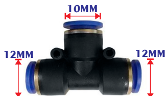
UNIÃO "T" PARA EMENDA C/ REDUÇÃO 12MM X 10MM
