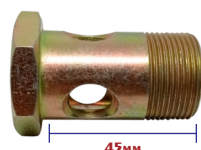
PARAFUSO OCO DO CANO DO COMPRESSOR 26MM
