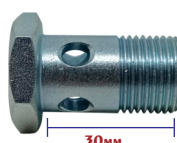
PARAFUSO OCO M18 X 1,5MM
